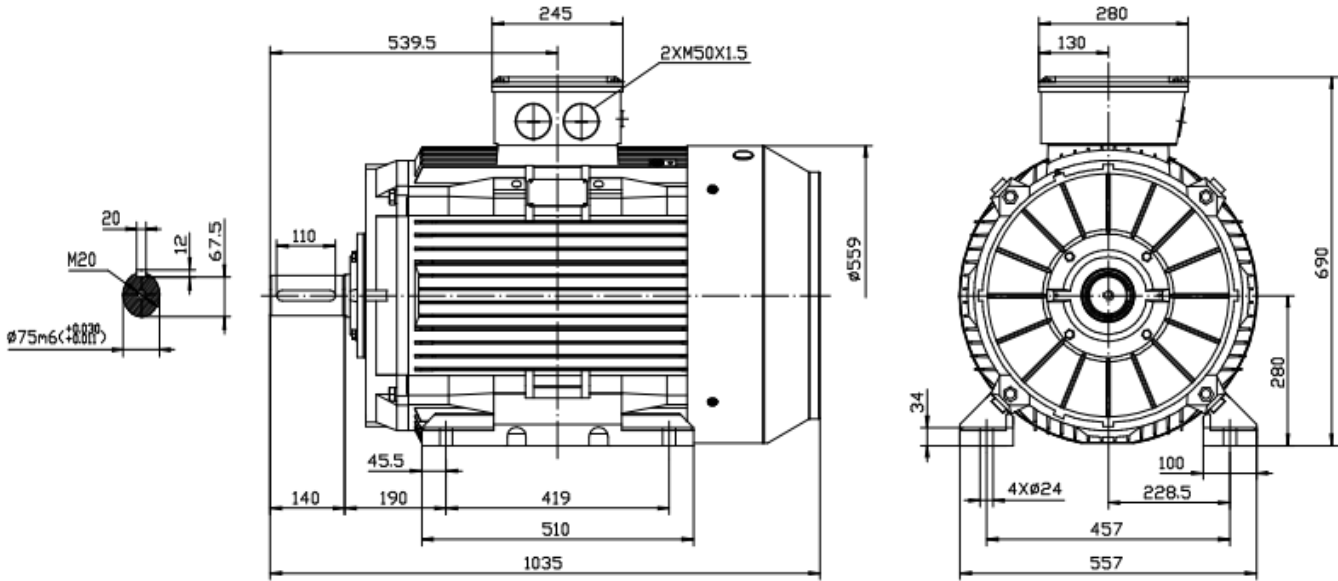
Typ / type IE3 SEV- 280M-8
