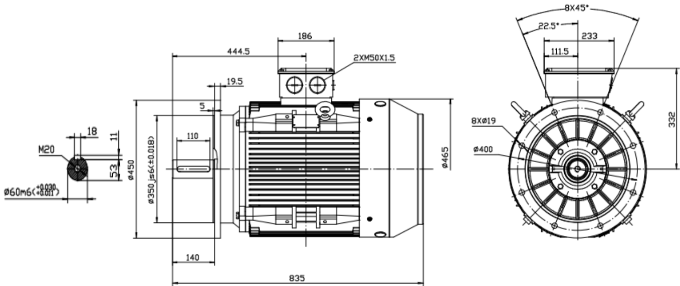
Typ / type IE3 SEV- 225M-8
